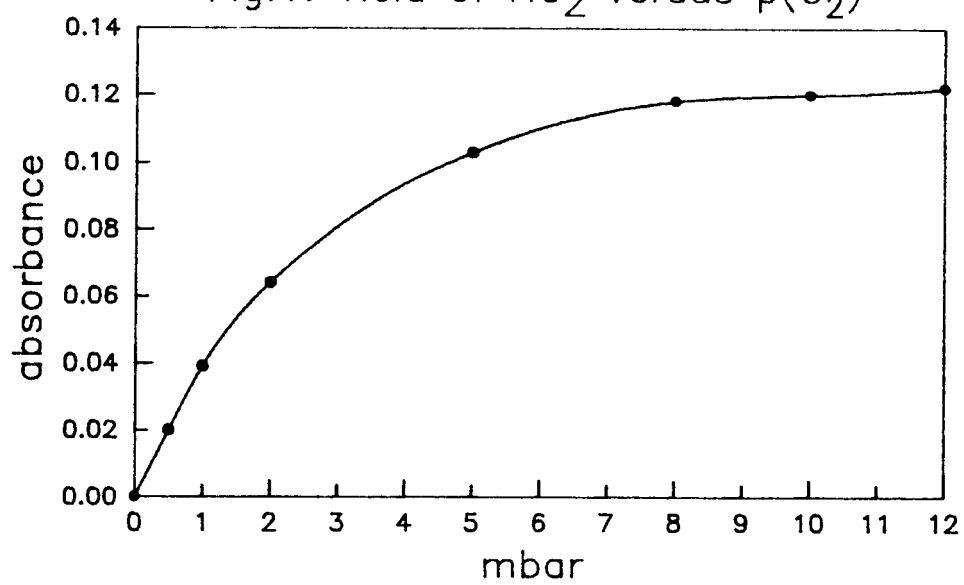
Fig.1. Yield of HO 2 versus p(O 2 )
